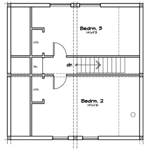
Optional Loft Floor Plan
